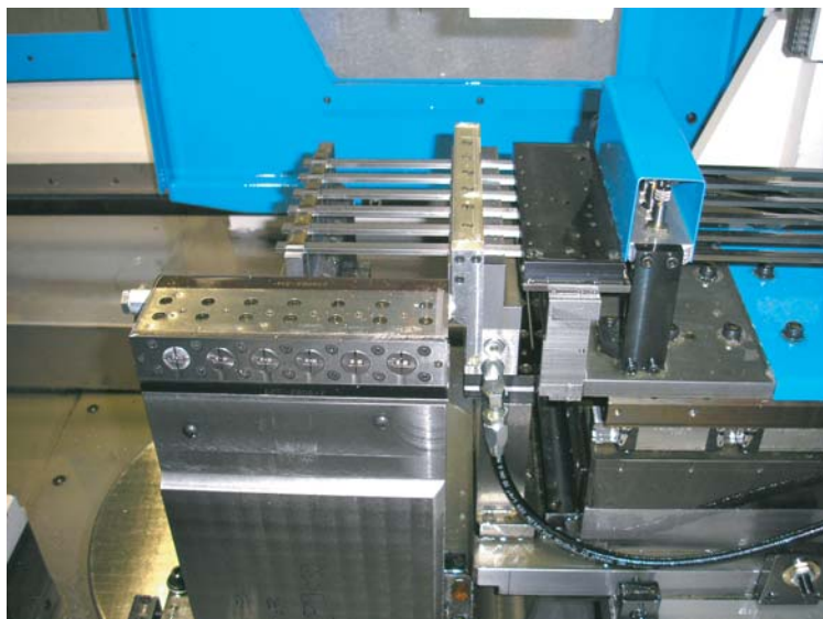
Avance barres
