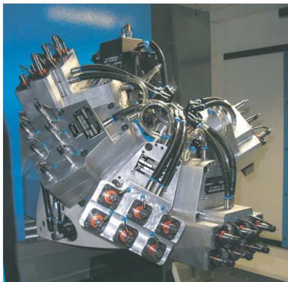
Station d'usinage
